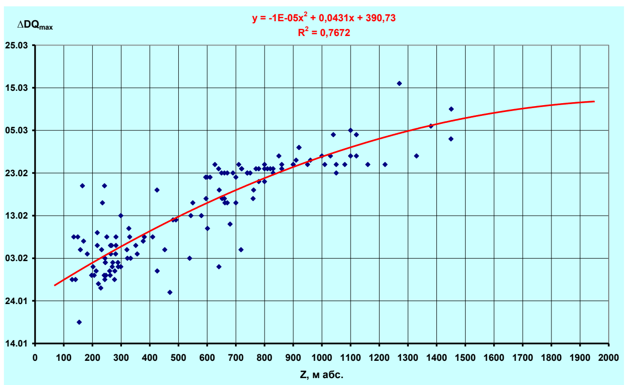
Рис. 21. Залежність середніх дат максимальних запасів снігу ( \bar{D} Q_{\max} ) імовірності від висоти, за даними спостережень на південному (а) та північному (б) макросхилах регіону
