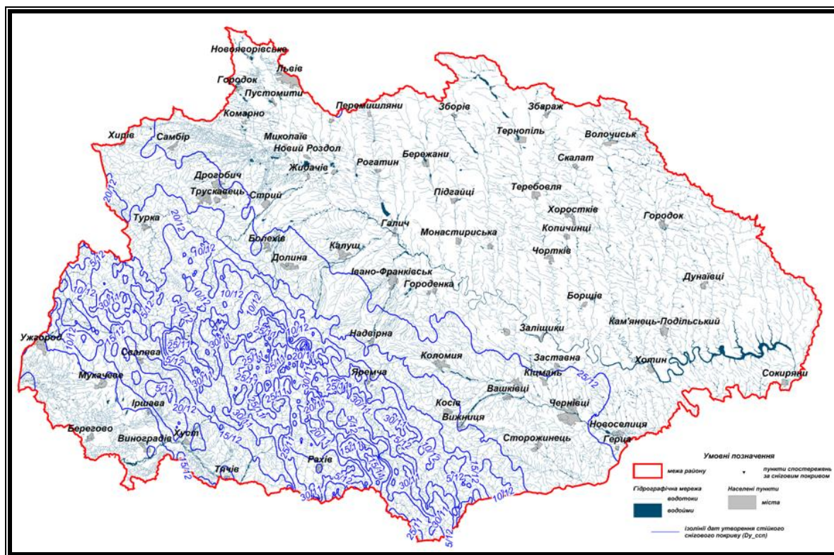
Рис.9. Дати утворення стійкого снігового покриву ( D_y \text{ csp} )
