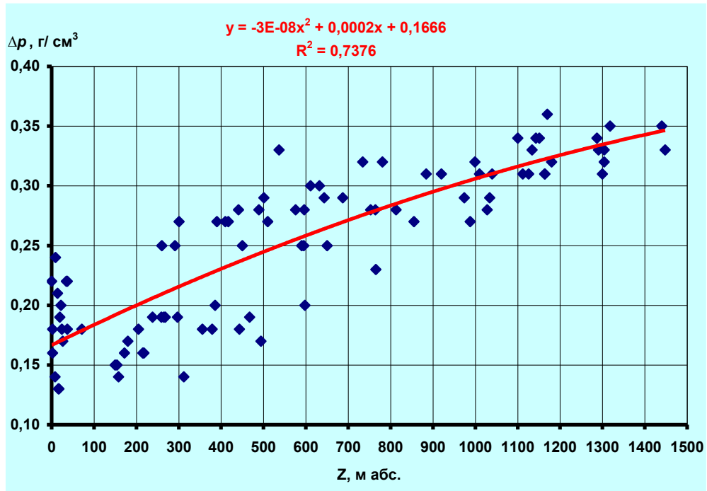
Рис. 9. Залежність середньої щільності снігу ( \overline{\rho} , г/см³) від висоти місцевості на південному (а) та північному (б) макросхилах регіону
