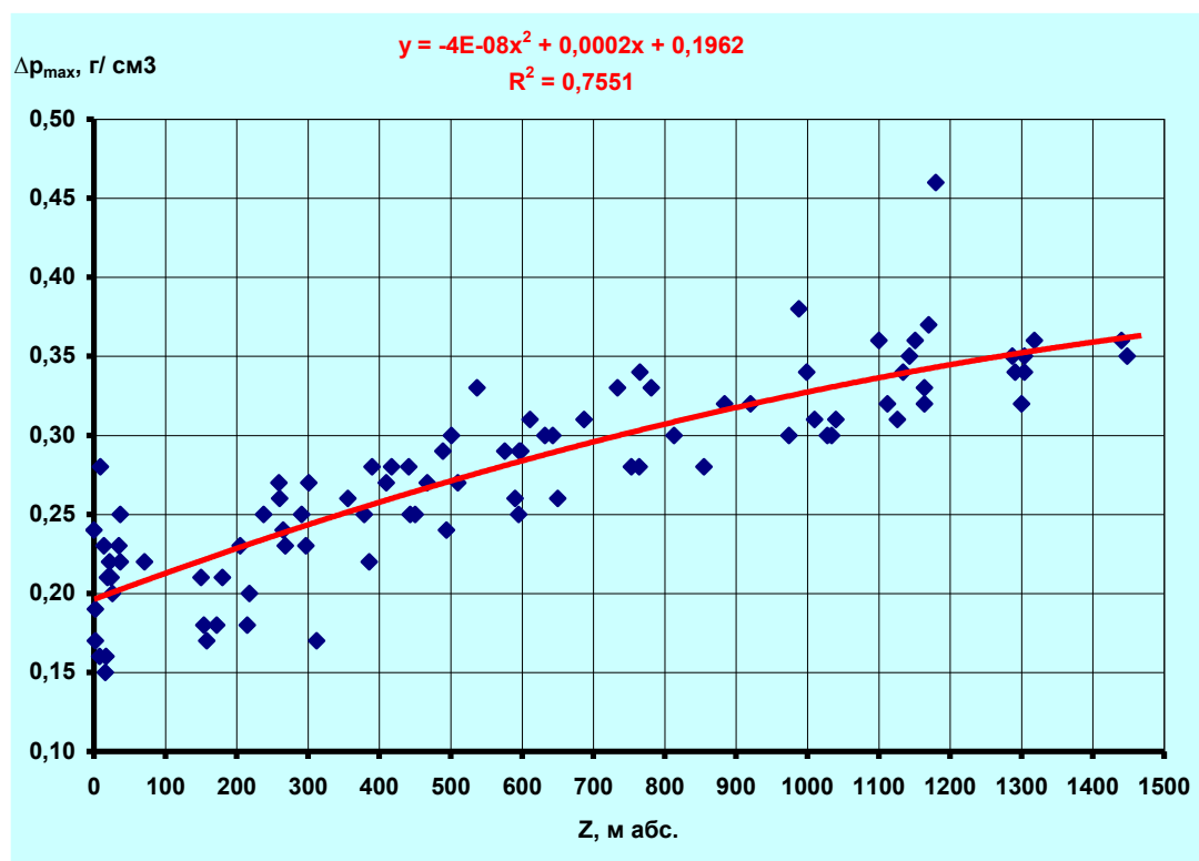
Рис. 10. Залежність середньої максимальної щільності снігу ( \bar{\rho}_{\max} , g/cm³) від висоти місцевості на південному (а) та північному (б) макросхилах регіону
