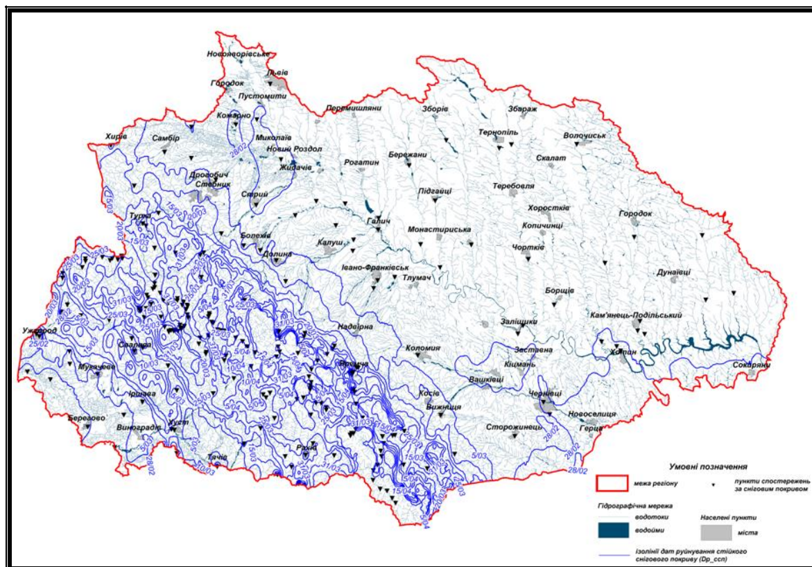
Рис.10. Дати руйнування стійкого снігового покриву ( D_r \text{ csp} )
