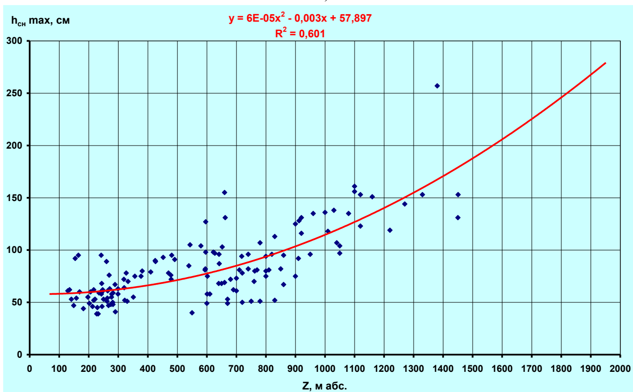
Рис. 18. Залежність максимальної висоти снігового покриву ( h_{ch} \text{ max, см} ) від висоти, за даними спостережень на південному (а) та північному (б) макросхилах регіону
