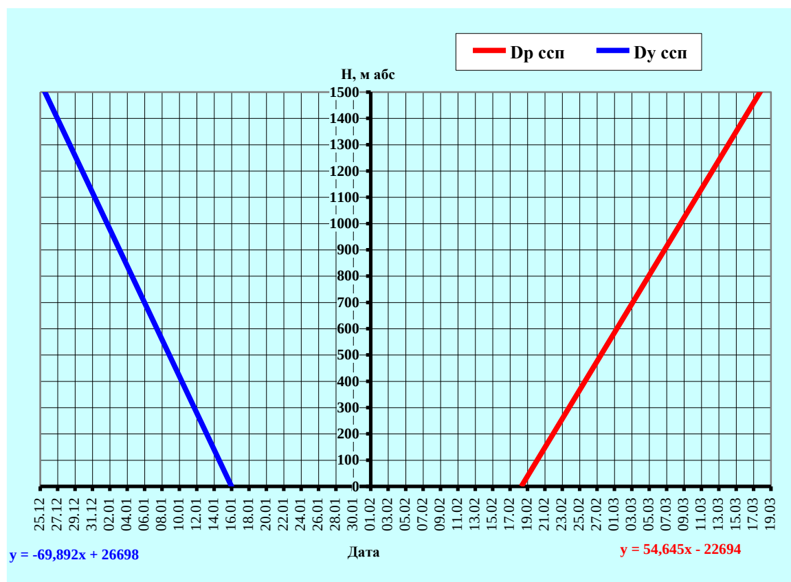
Рис.2.6 Обчислена залежність середніх багаторічних дат утворення (Du) та руйнування (Dp) стійкого снігового покриву від висоти на північному макросхилі Кримських гір
