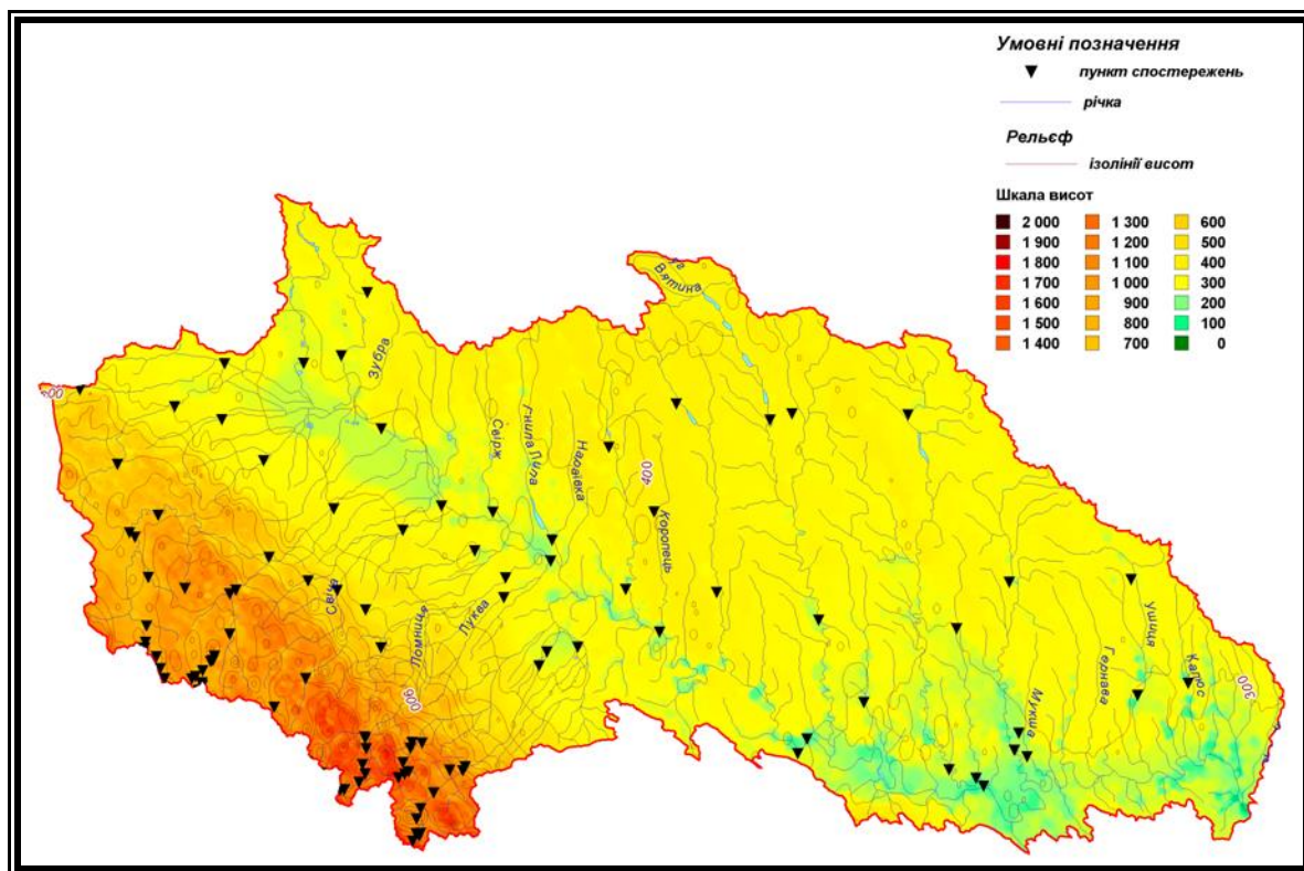
Рис.5. Басейн р. Дністра
