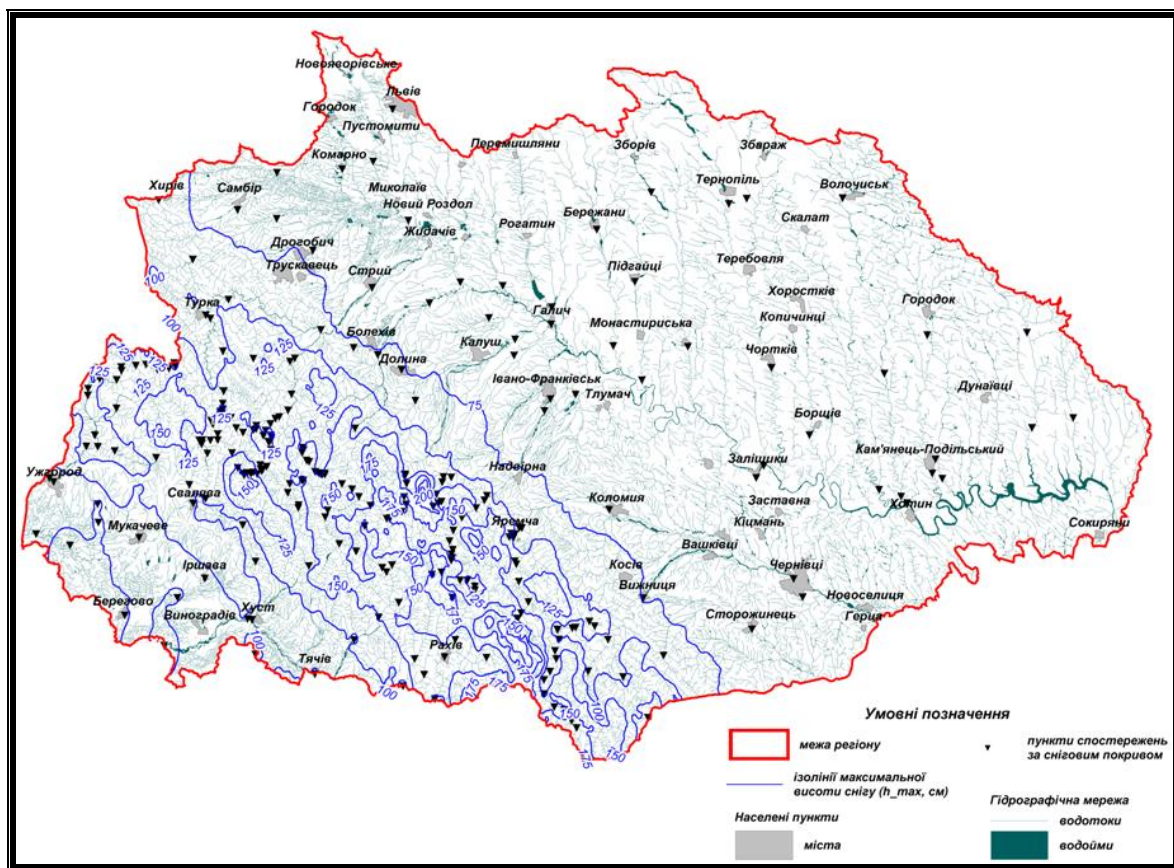
Рис.11. Максимальна висота снігу ( h_{ch\_max} )
