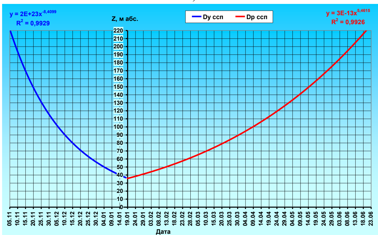
Рис. 17. Залежність кількості днів із стійким сніговим покривом ( N_{ccn} ) від дат утворення ( Dy ) та руйнування ( Dp ) стійкого снігового покриву, за даними розрахунків, від висоти місцевості на південному (а) та північному (б) макросхилах регіону
