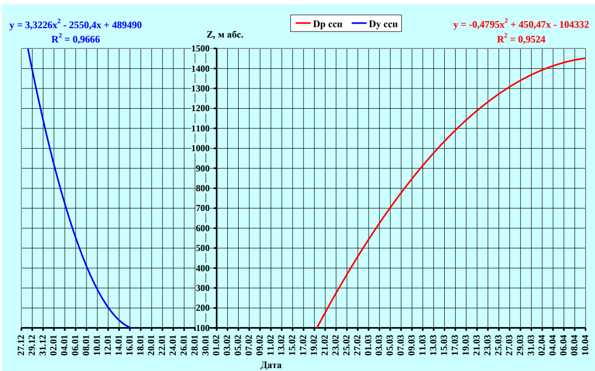
Рис. 17. Залежність дат утворення ( Dy ) та руйнування ( Dp ) стійкого снігового покриву, за даними розрахунків, від висоти місцевості на південному (а) та північному (б) макросхилах регіону
