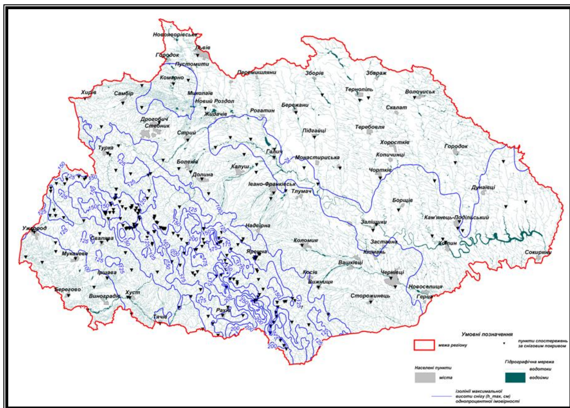
Рис.12. Максимальна висота снігу ( h_{ch\_max} ) 1% імовірності
