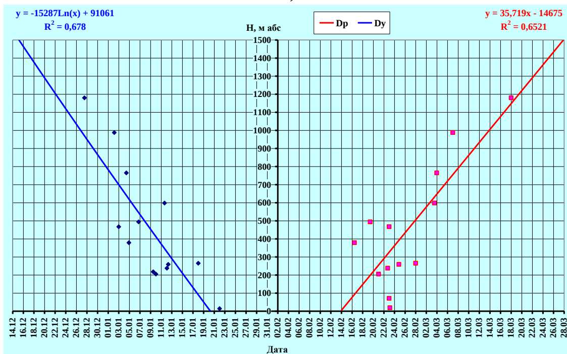
Рис. 16. Залежність дат утворення (Dy) та руйнування (Dp) стійкого снігового покриву, за даними спостережень, від висоти місцевості на південному (а) та північному (б) макросхилах регіону за даними спостережень.
